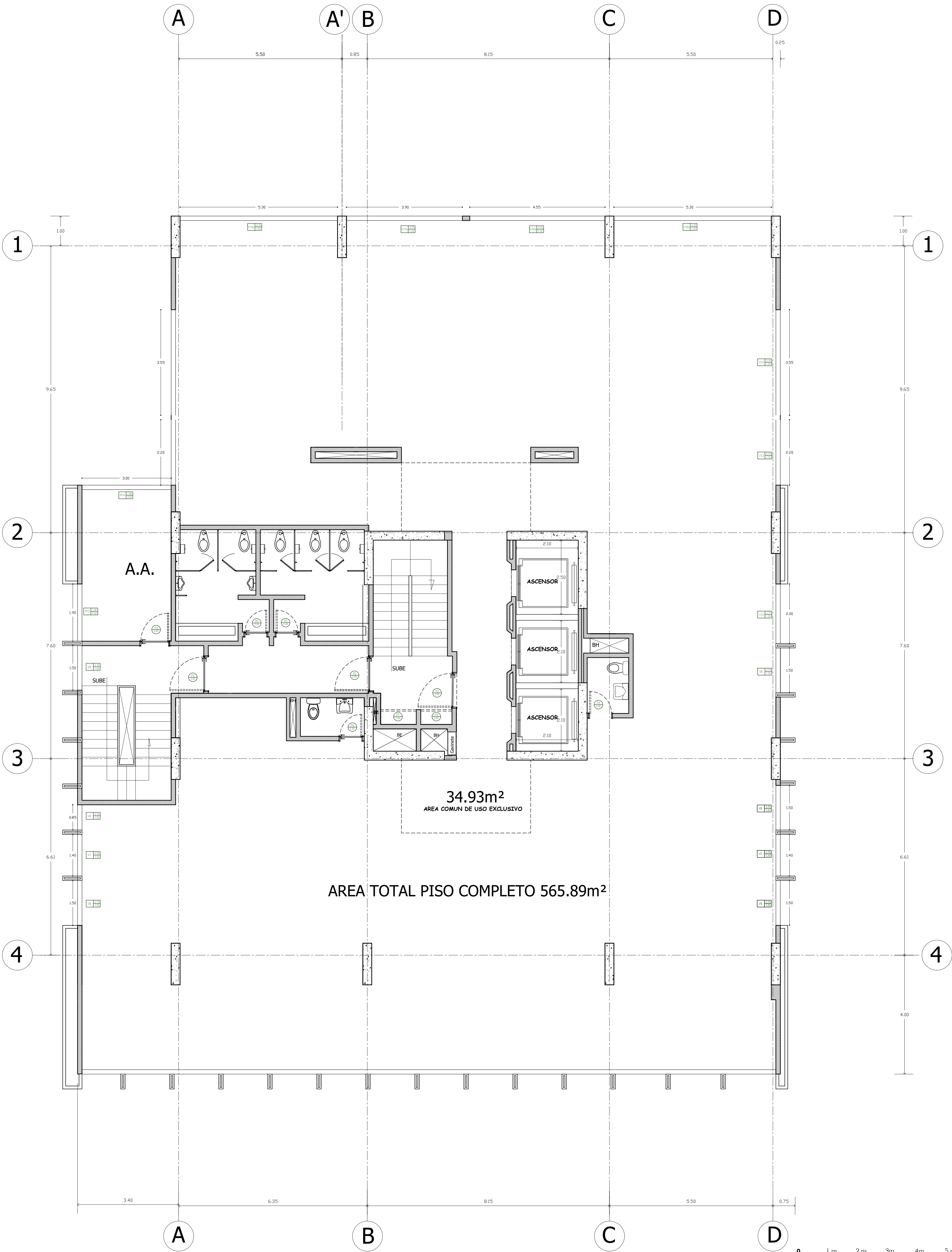
PLANTA TIPO OPCION PISO COMPLETO
